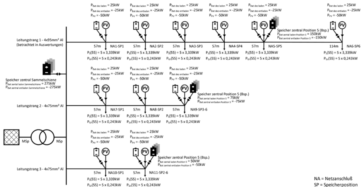
Abbildung 3: Schema Referenznetz mit 11 Netzanschlüssen (55 Hausanschlüssen) inkl. PV-Anlagen und zentralen/dezentralen Speichersystemen, Quelle: eigene Darstellung
